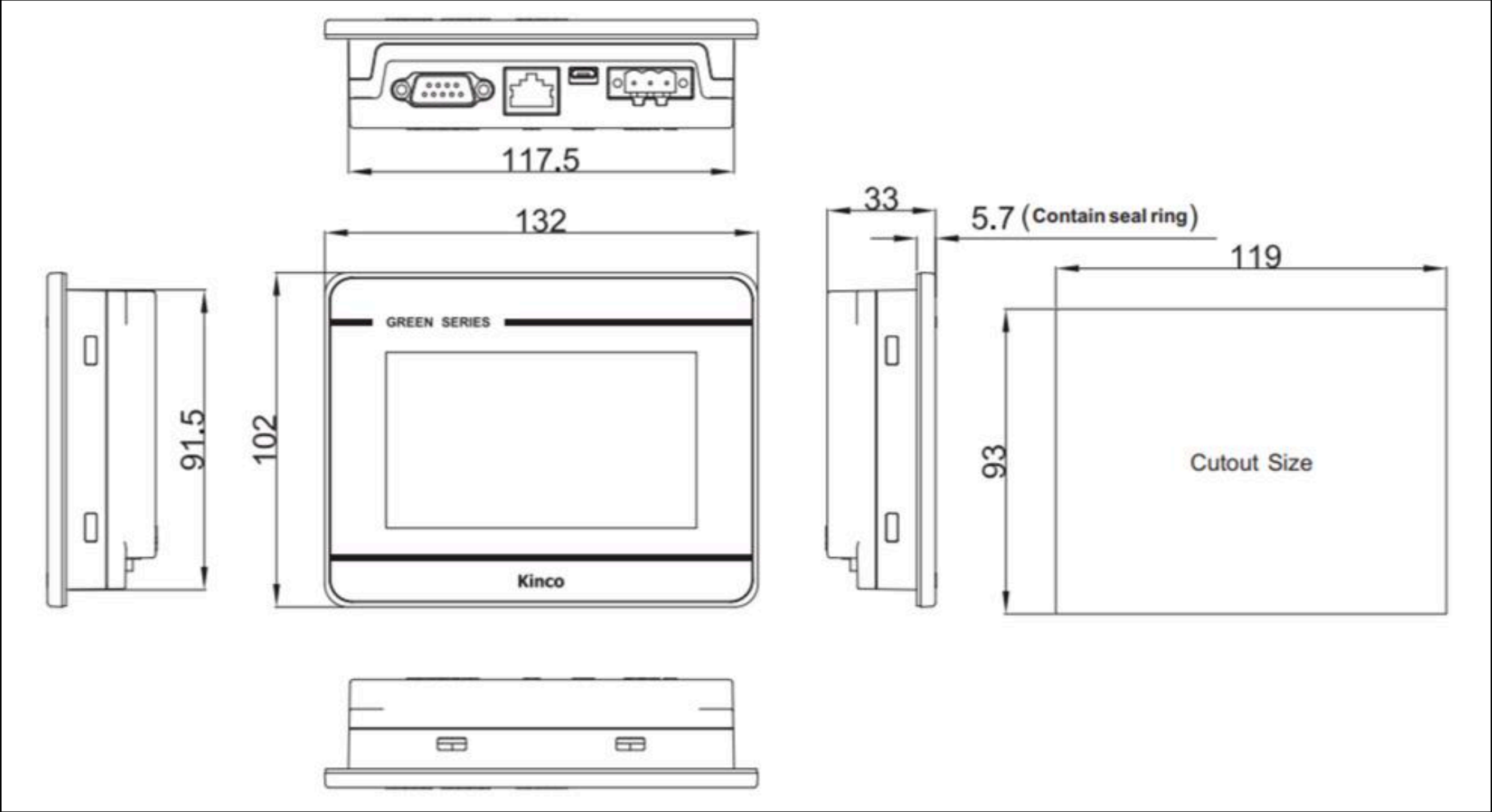
Рисунок 1 - Габаритные и посадочные размеры GL043, GL043E
