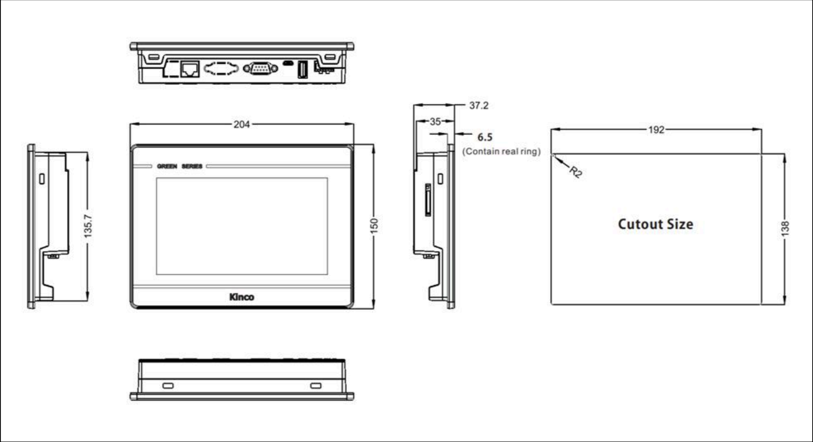
Рисунок 2 - Габаритные и посадочные размеры GL070, GL070E
