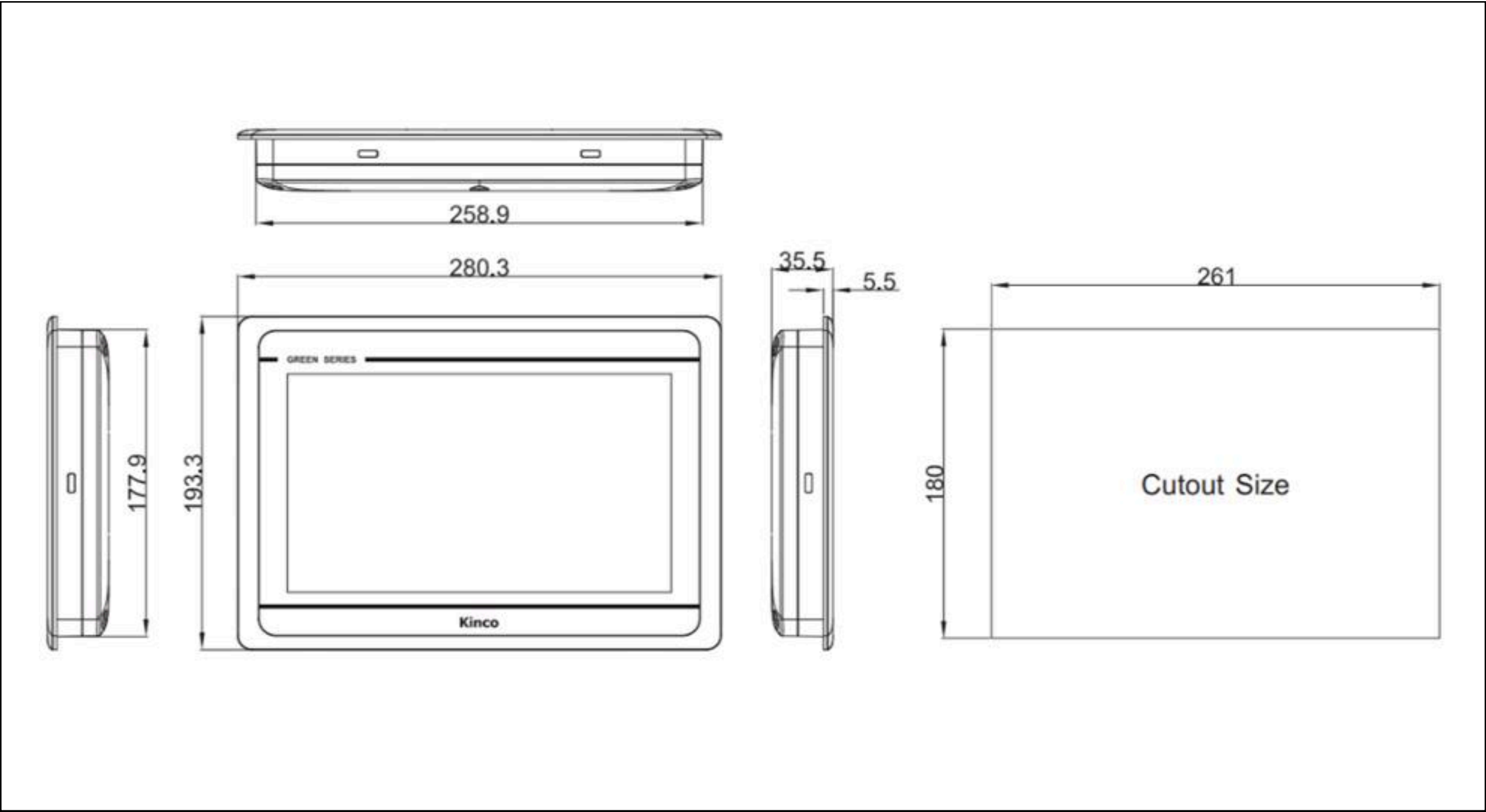
Рисунок 3 - Габаритные и посадочные размеры GL100, GL100E
