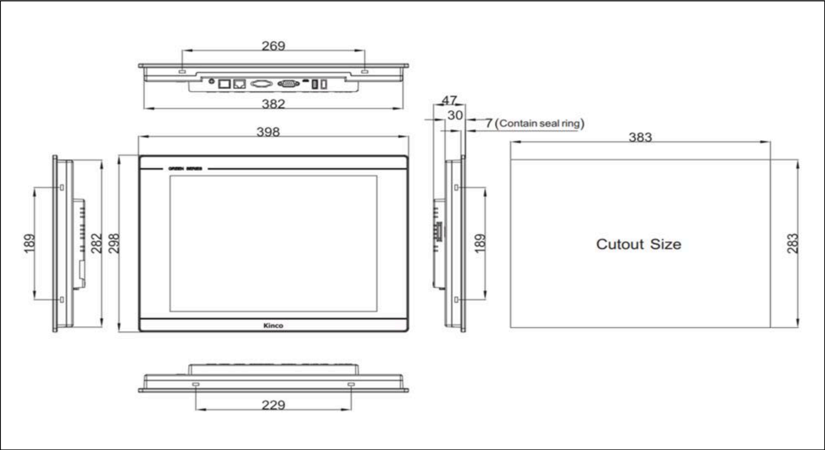
Рисунок 4 - Габаритные и посадочные размеры GL150E
